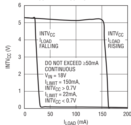
\text{INTV}_{\text{CC}} vs \text{INTV}_{\text{CC}} I_{\text{LOAD}}
